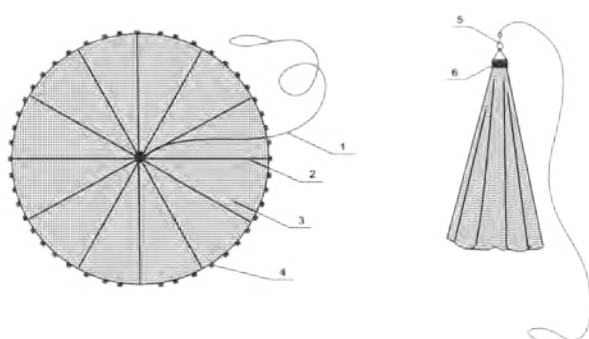
Рис. 3.27. Сіть «Парашут» або кастингова сітка: 1 – центральний тяговий шнур; 2 – стропи; 3 – полотно сітки; 4 – вантажний шнур; 5 – вертлюг; 6 – втулка
